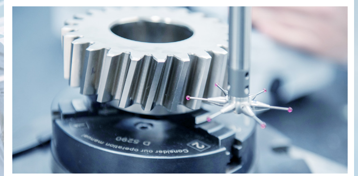
Pomiary kół zębatych
